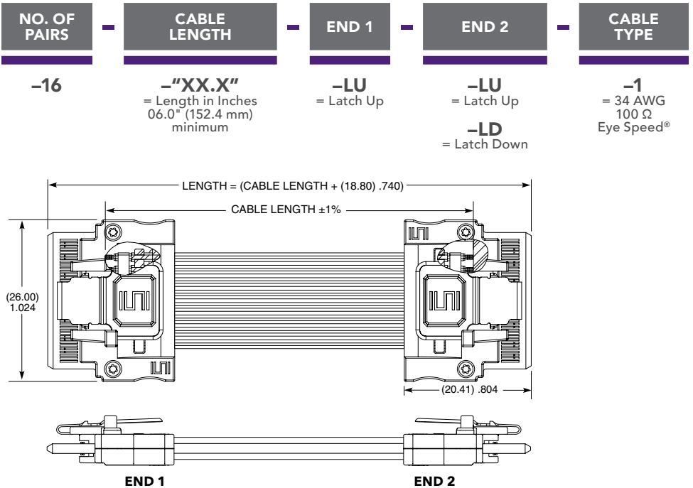
FEDP-16-XX.X-LU-LU-1 SHOWN
