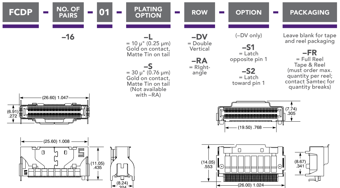
FCDP-16-01-X-DV-S1 SHOWN
