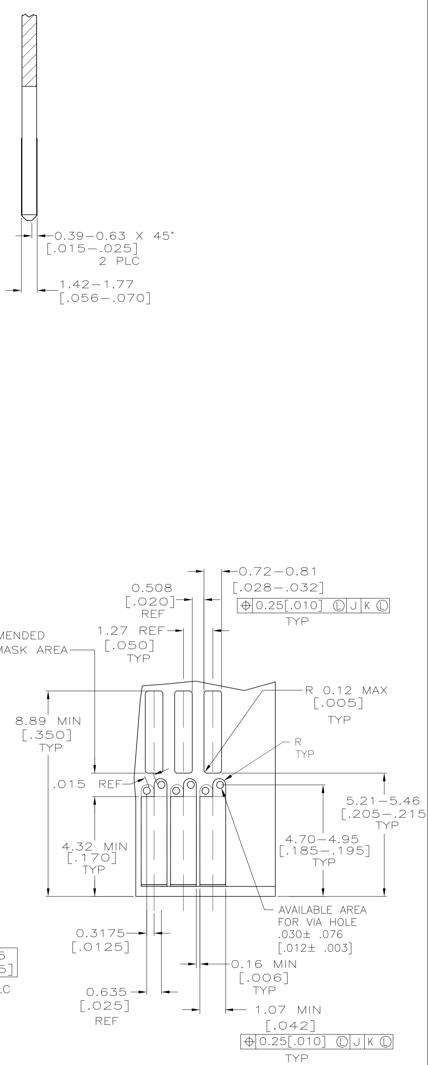
DETAIL H SCALE: 10 : 1
