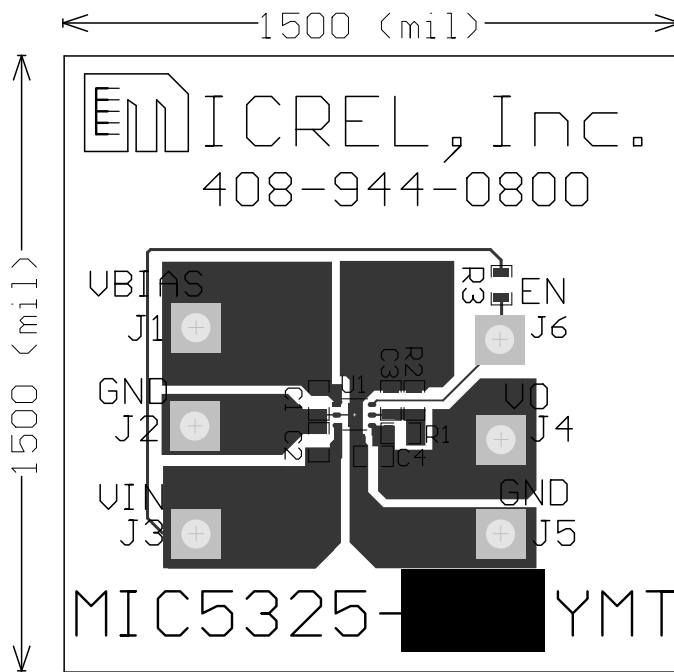
Top Layer
