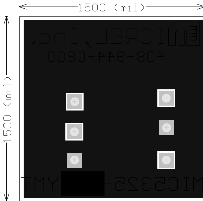
Bottom Layer
