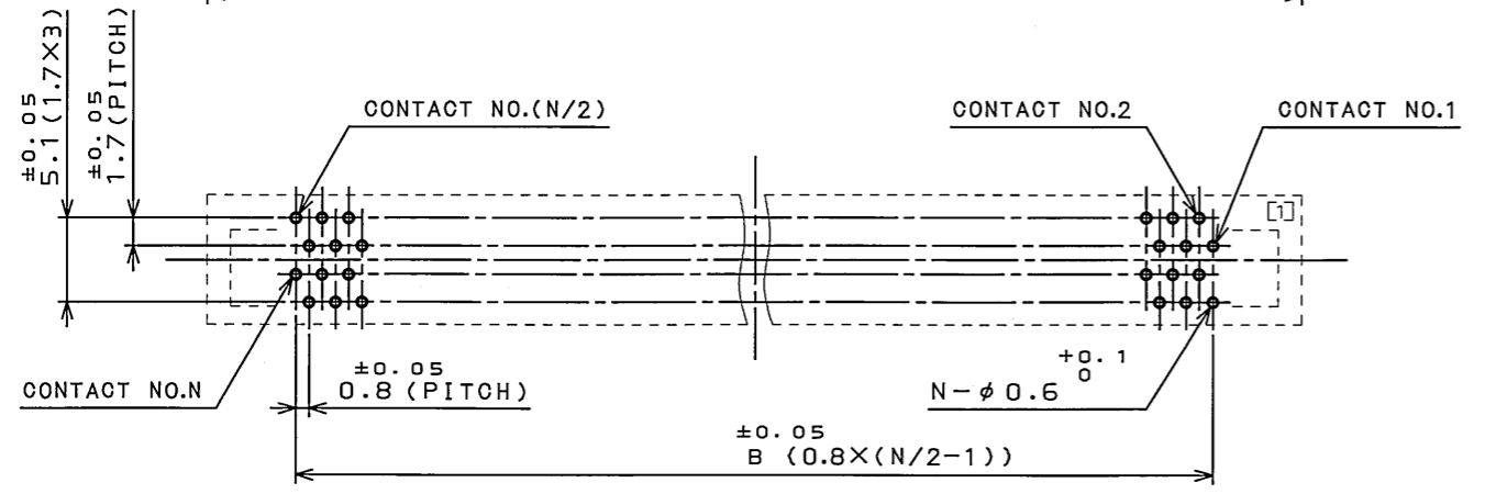
P.C.B. HOLE PATTERNS (REF.) 基板取付穴寸法 (参考)
