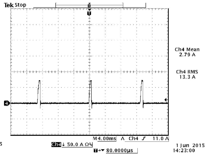
Vin=12V, Vo=0.9V
