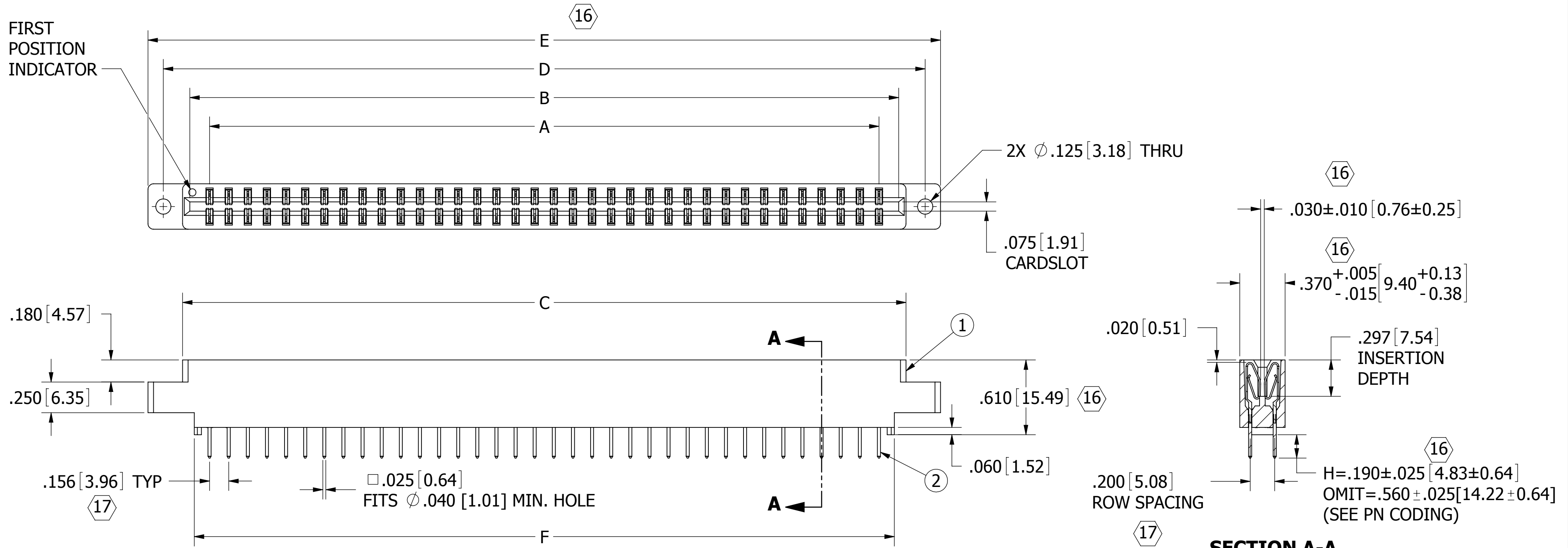
SECTION A-A SCALE 2 : 1.25
