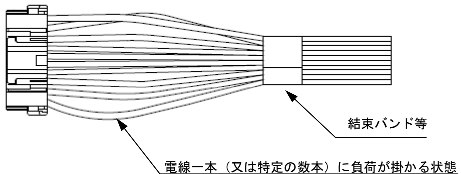
Fig.7-2 不適切なハーネス結束状態
