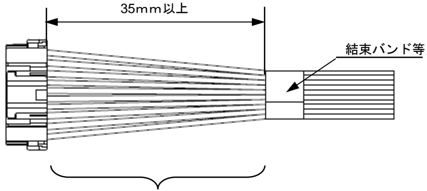
Fig.7-1 適切なハーネス結束状態
