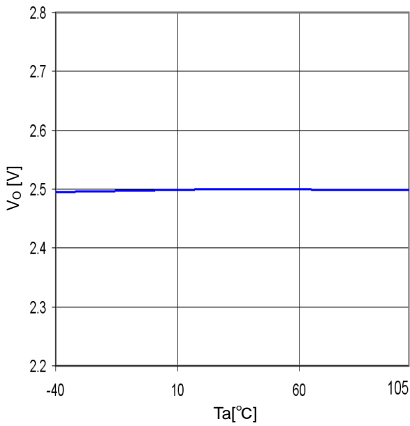
Figure 21. Ta-V o (I o =0mA)
