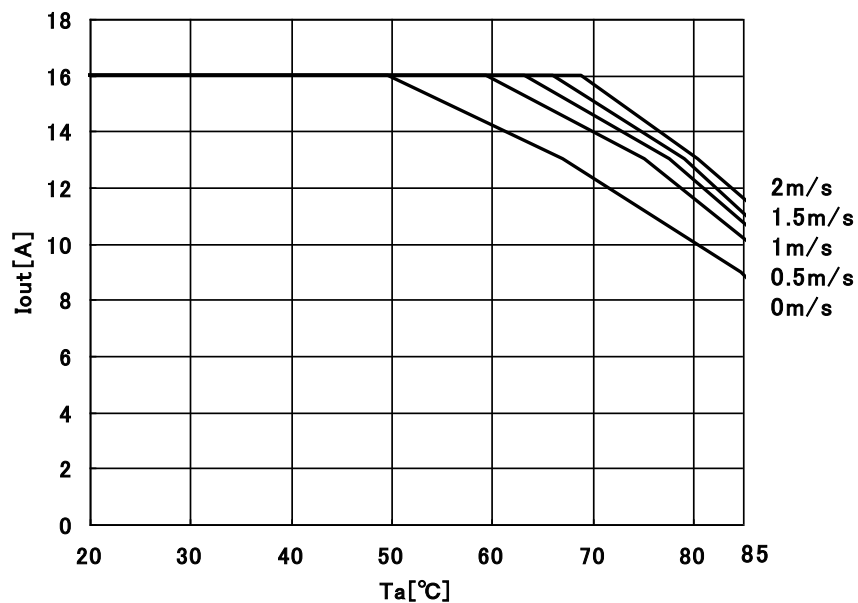
Thermal Derating (MPD TY312S)
