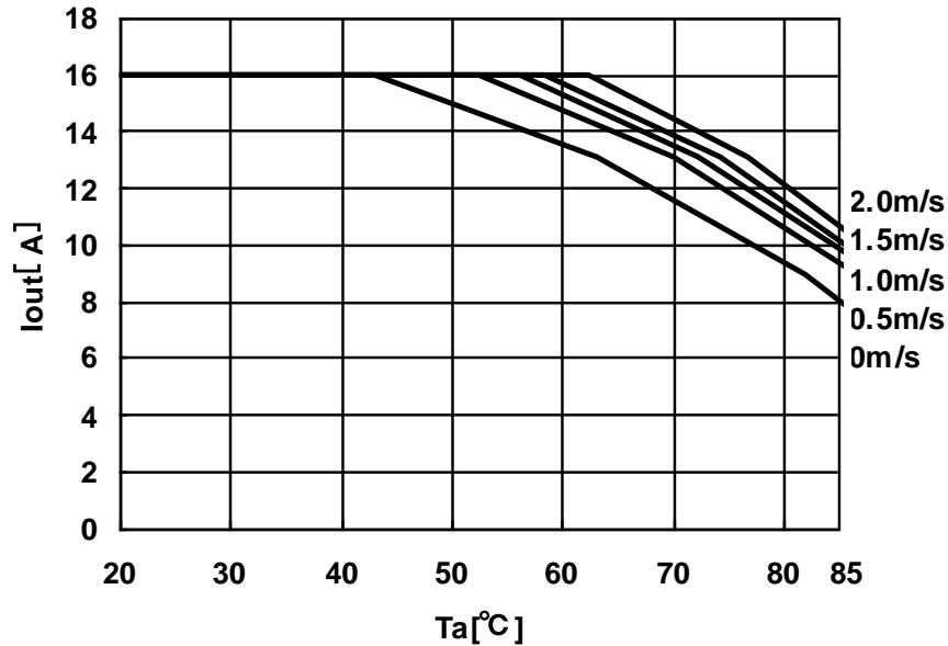
Thermal Derating (MPD TY311S)
