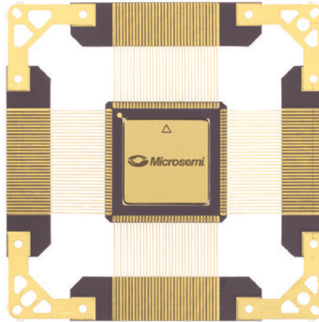
CQ132 b.s. 0.95" x 0.95" (24.13 mm x 24.13 mm) h. 105 mils (2.67 mm) p. 25 mils (0.64 mm)
