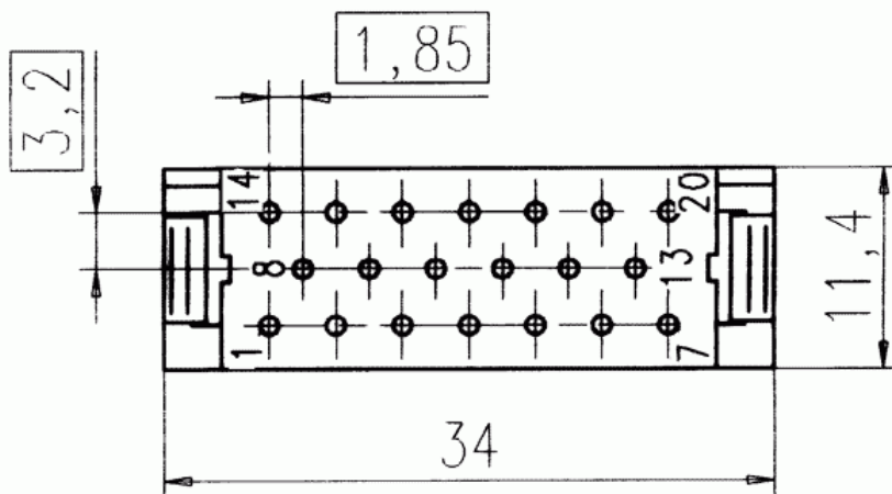
Maßzeichnung Dimensions in mm (Inch)
