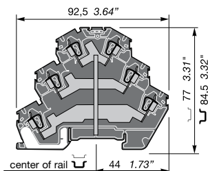
D 2,5/5.T1.L
