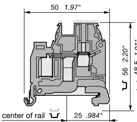
D 4/6.P.ADO
