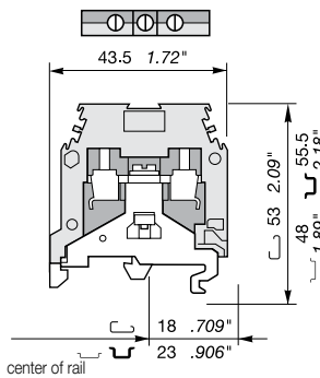
M 4/6.P
