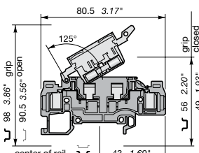
D 1,5/8.SNNT.ADO
