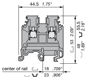
M 4/6
