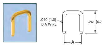
.040 (1.0) PINS
