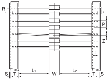
アキシャルテーピング Axial taping
