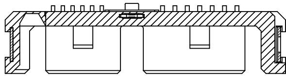
SECTION D-D
