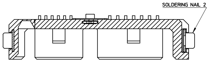
SECTION D-D
