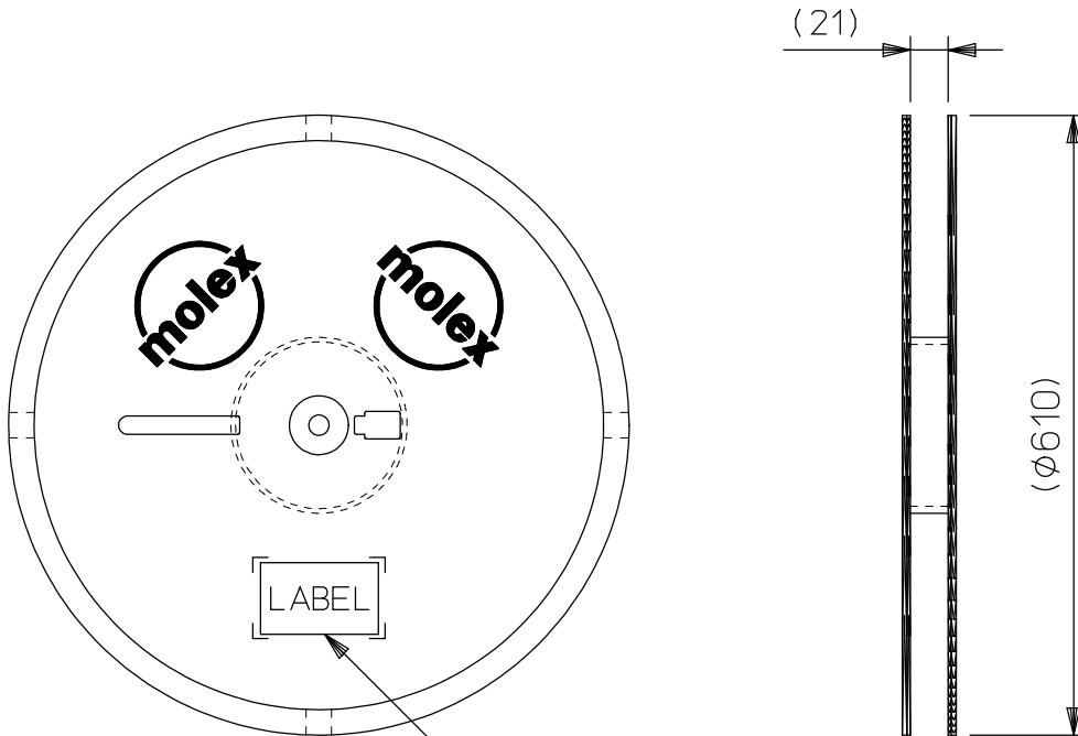
現品票 PART IDENTIFICATION LABEL (製品型番, 数量, ロットNO. 表示) INDICATION OF PART No., QUANTITY, LOT No.
