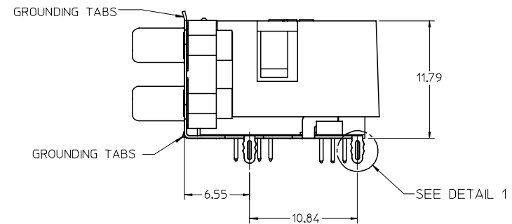
PRESS FIT FORKLOCK SHOWN (VERSION 4)
