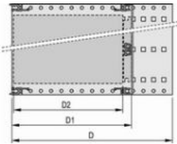
D=total depth, D1=insertion depth, D2=board depth
