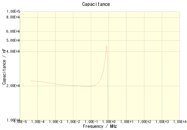
C3225X5R1A226M230AA
