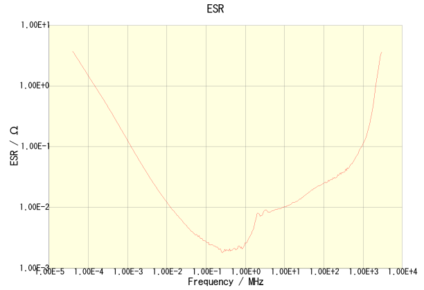
C3225X5R1A226M230AA
