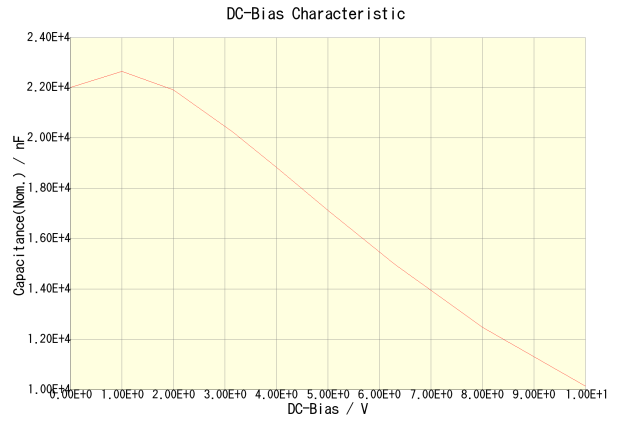
C3225X5R1A226M230AA
