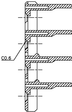
SECT A-A
