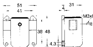
Montageausschnitt/Panel cut-out ø 20
