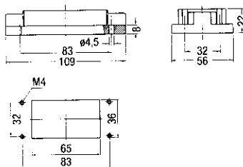
Montageausschnitt/Panel cut-out
