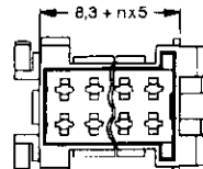
Flachstecker-Gehäuse/Tab Housing
