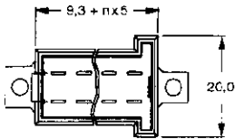
180°-Messerleiste/Pin Header 180°
