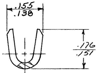
VIEW A-A
