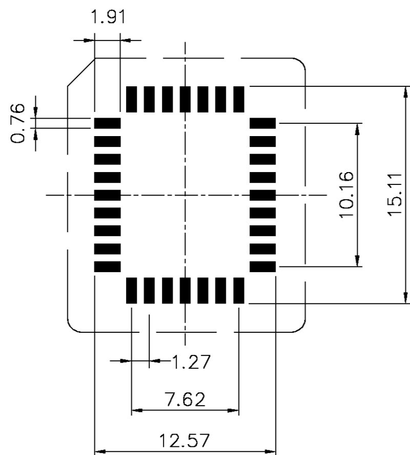
P.C.B. LAYOUT
