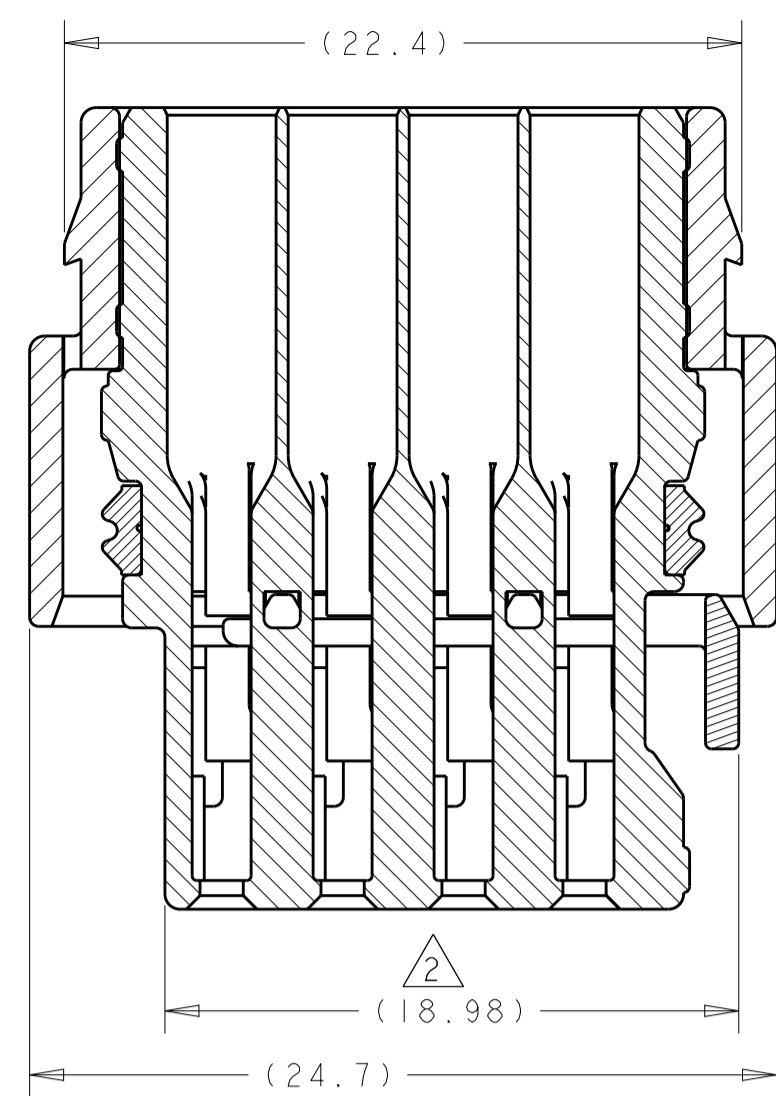
SECTION A-A
