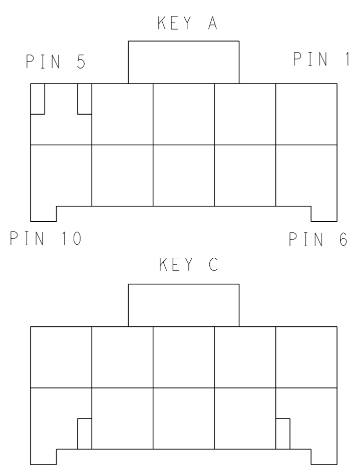
KEYING FOR 2*5 POS.
