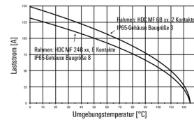
HDC-MHP100-Module im IP65-Gehäuse, Leiter HO7V-K35:
