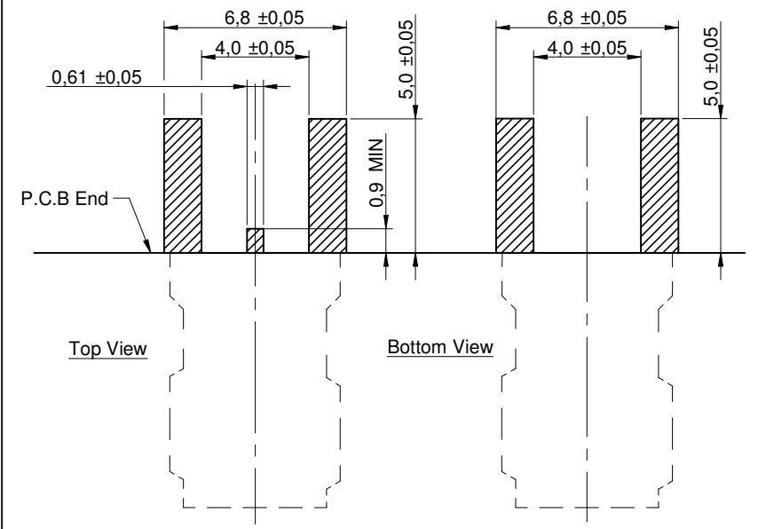
P.C.B Thickness: 1,6 mm
