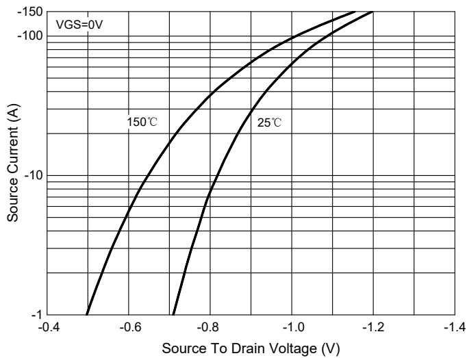
Fig.9 - I_s - V_{SD}
